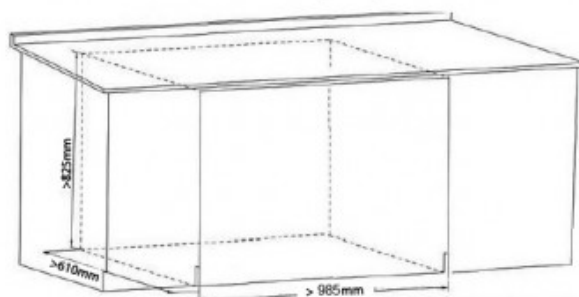
Instalação módulo Duplo (Charutos + Vinho)
